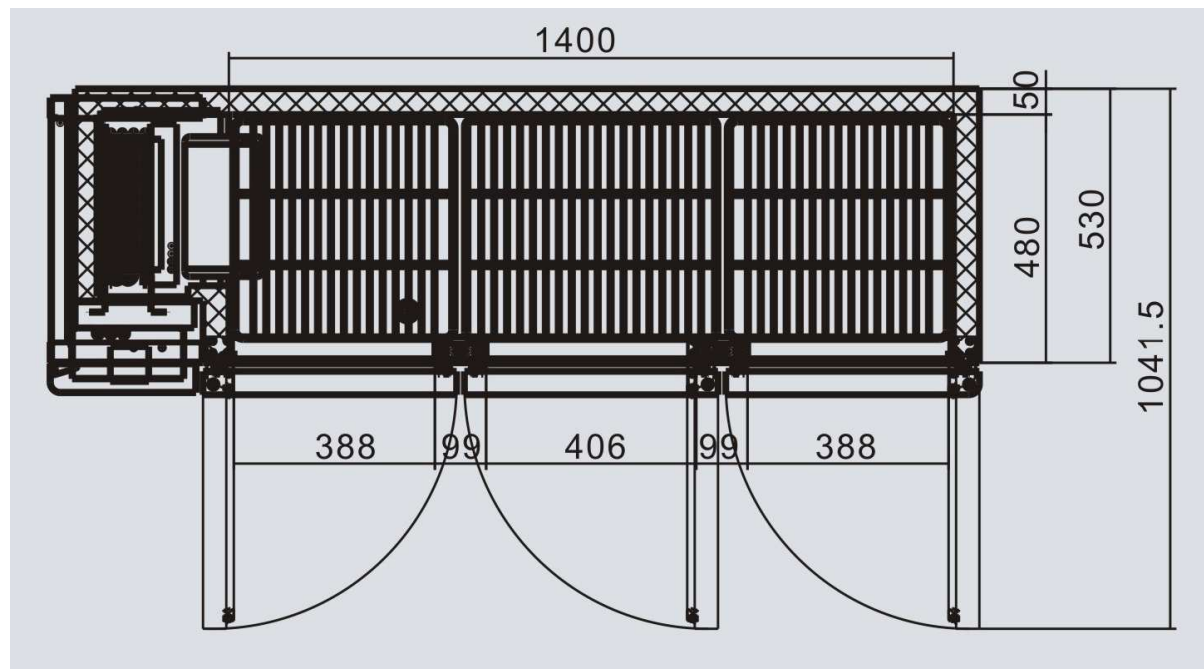
Rys.2. Stół chłodniczy Kitchen Line 3-drzwiowy, z agregatem bocznym, linia 600 – z góry
