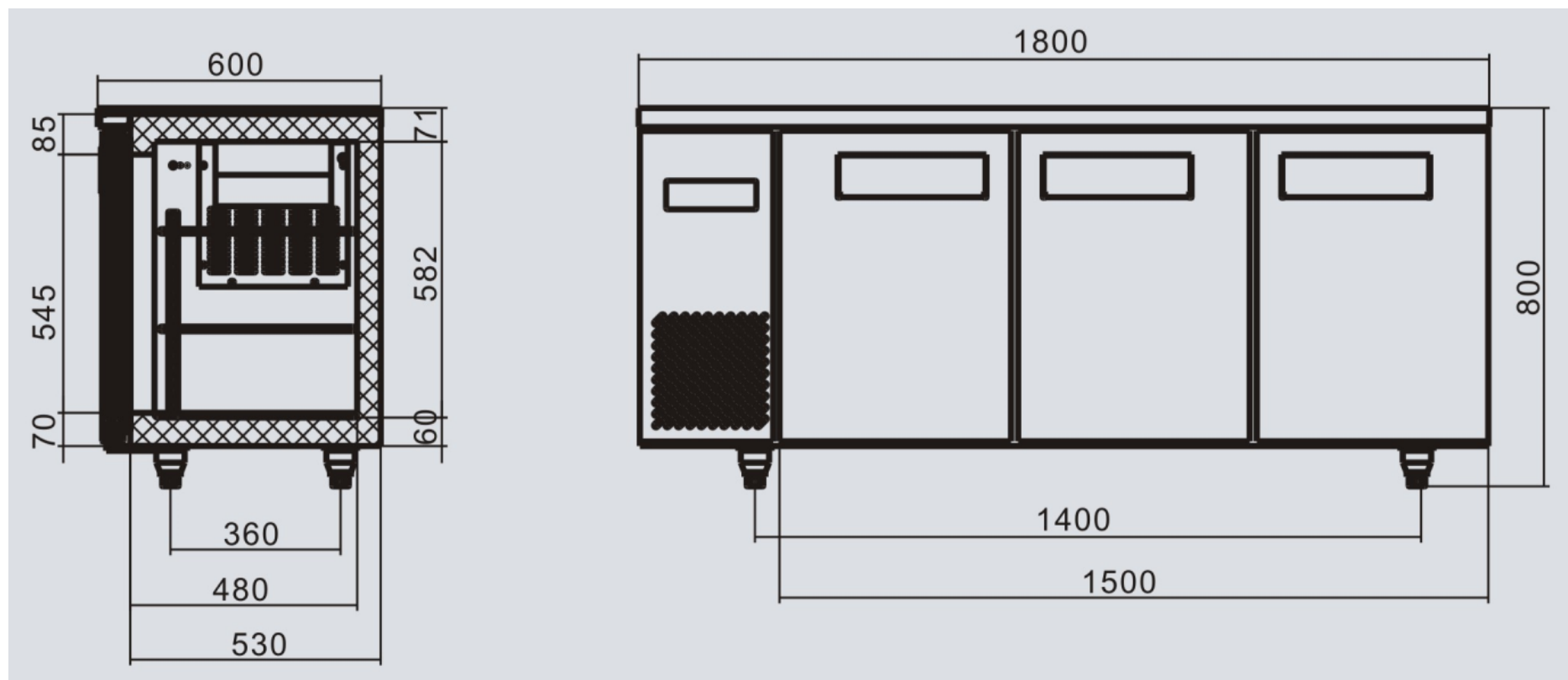
Rys.1. Stół chłodniczy Kitchen Line 3-drzwiowy z agregatem bocznym, linia 600 –widok z boku (po lewej) oraz z przodu (po prawej)
